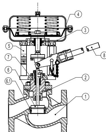
VPA26S– с пневматическим приводом и ручным управлением
