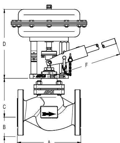
VPA26S– с пневматическим приводом и ручным управлением
