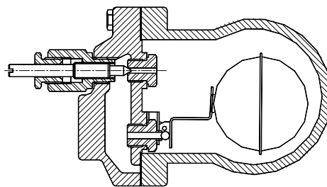
FLT16 DN15-20
