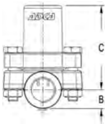
ГАБАРИТНЫЕ РАЗМЕРЫ (mm)
